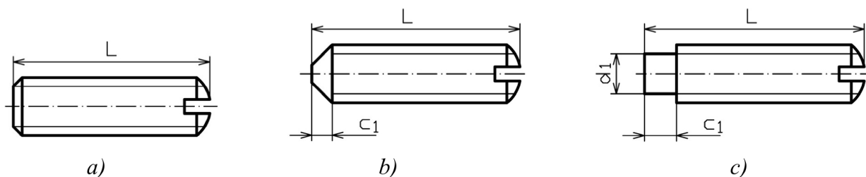
Sl.11.22. Osnovne dimenzije uvrtnih zavrtnjeva: a) bez završetaka, b) sa šiljkom, c) sa cilindričnim završetkom
